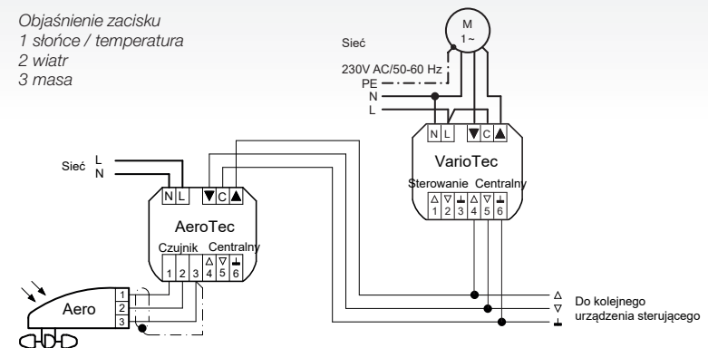
Rysunek podłączenia do sterowania grupowego lub centralnego
