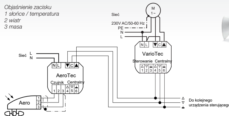
Rysunek podłączenia do sterowania grupowego lub centralnego
