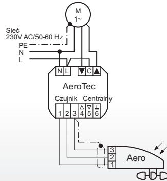
Indywidualna kontrola - rysunek połączenia
