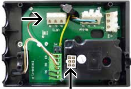
sechs-poliger Stecker Steuerung Anschlußkabel
