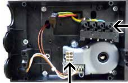
Fiche à six pôles Câble de connexion de commande
