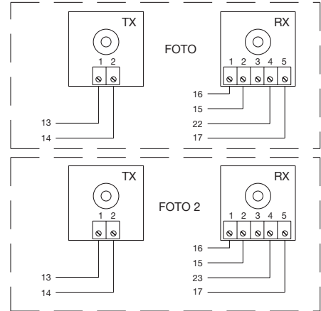
Fig. 3A Conexión fototest con las fotocélulas "Fotocélula" y "Fotocélula 2"
