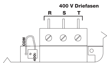
Aansluiting van de besturingseenheid met een stroomtoevoer 400V driefasen
