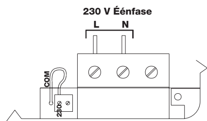
Aansluiting van de besturingseenheid met een stroomtoevoer 230V driefasen
