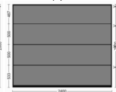
Bramy E120 – wykonanie opcjonalne (wym. spec.) Bramy ze sprężynami skrętnymi - standardowe wykonanie - panel ścięty symetrycznie do dolnego i okuty profilem aluminiowym
