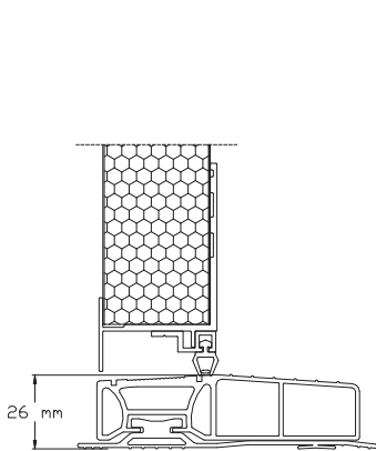
Próg 26 mm + uszczelka (bramy garażowe i przemysłowe)
