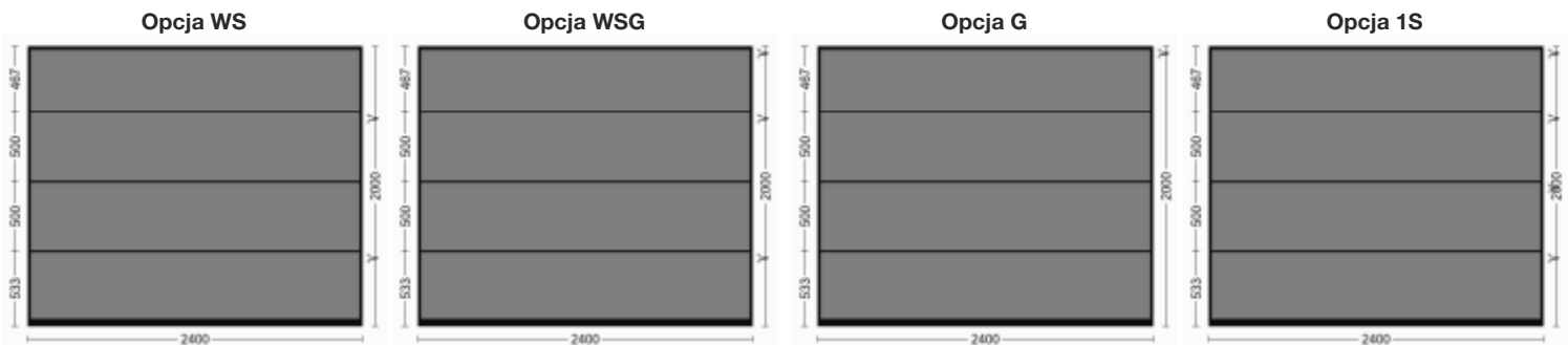
Bramy E120 – wykonanie opcjonalne (wym. spec.) Bramy ze sprężynami skrętnymi - standardowe wykonanie - panel ścięty symetrycznie do dolnego i okuty profilem aluminiowym
