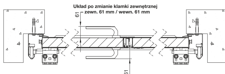
Układ po zmianie klamki zewnętrznej – zewn. 61 mm / wewn. 61 mm
