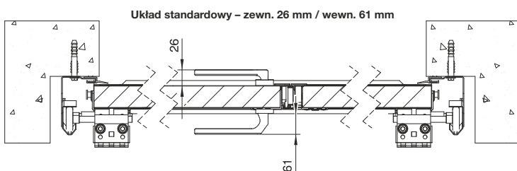
Układ standardowy – zewn. 26 mm / wewn. 61 mm
