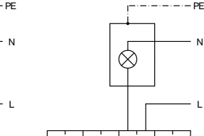
Sterowanie światłem
