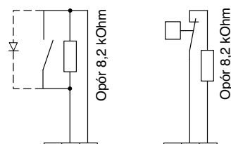
zacisk NO lub dioda LED zabezpieczenia przed zgnieciem Zabezpieczenie przed zgnieciem
