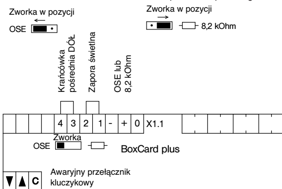
zacisk NO lub dioda LED zabezpieczenia przed zgnieciem Zabezpieczenie przed zgnieciem
