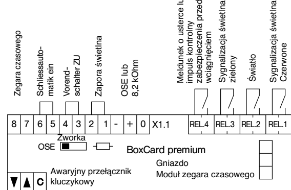
Włączanie/wyłączanie zegara czasowego
