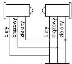
Zabezpieczenie przed zgnieciem OSE
